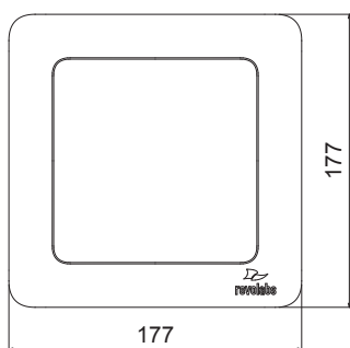
上面図
