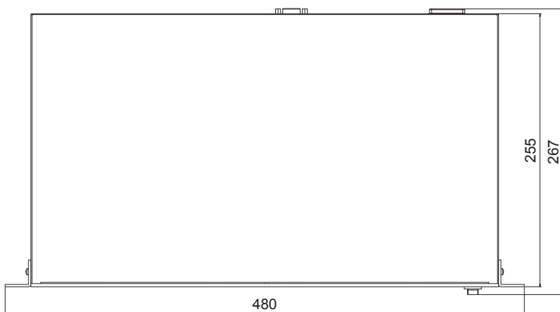
上面図
