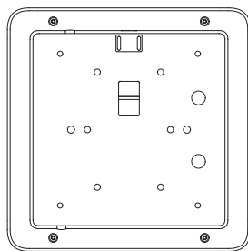
底面図
